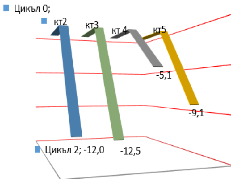
Фиг. 5. Диаграма на хоризонталните деформации между втория и нулевия цикъл
