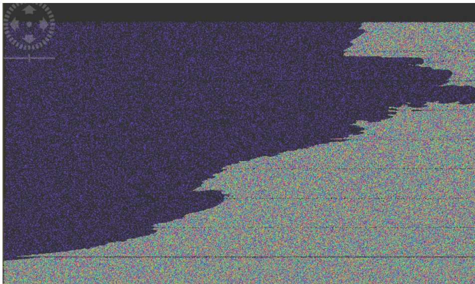
Фиг. 3. Интерферограма на района на изследване
