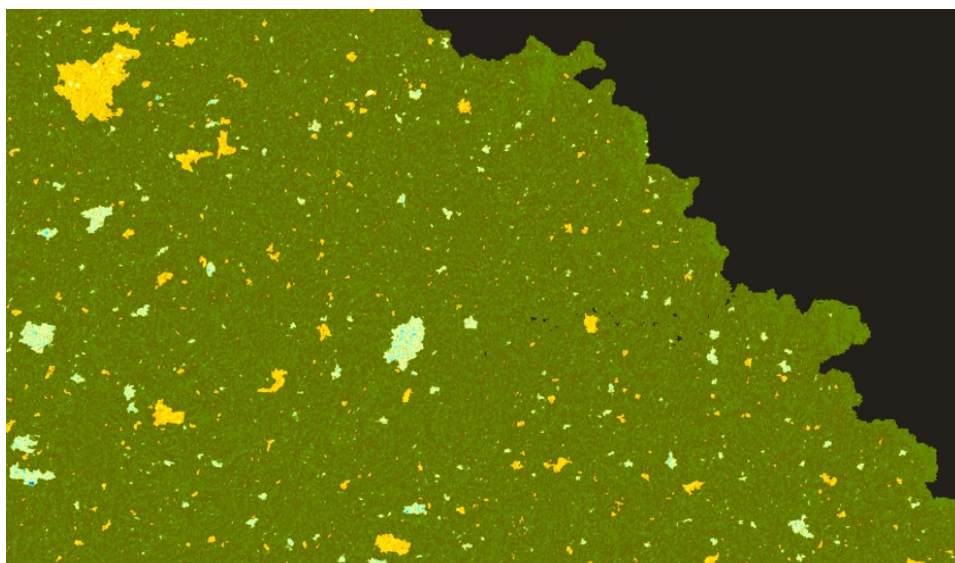
Фиг. 4. Относително изместване на земната повърхност в изследваната територия
