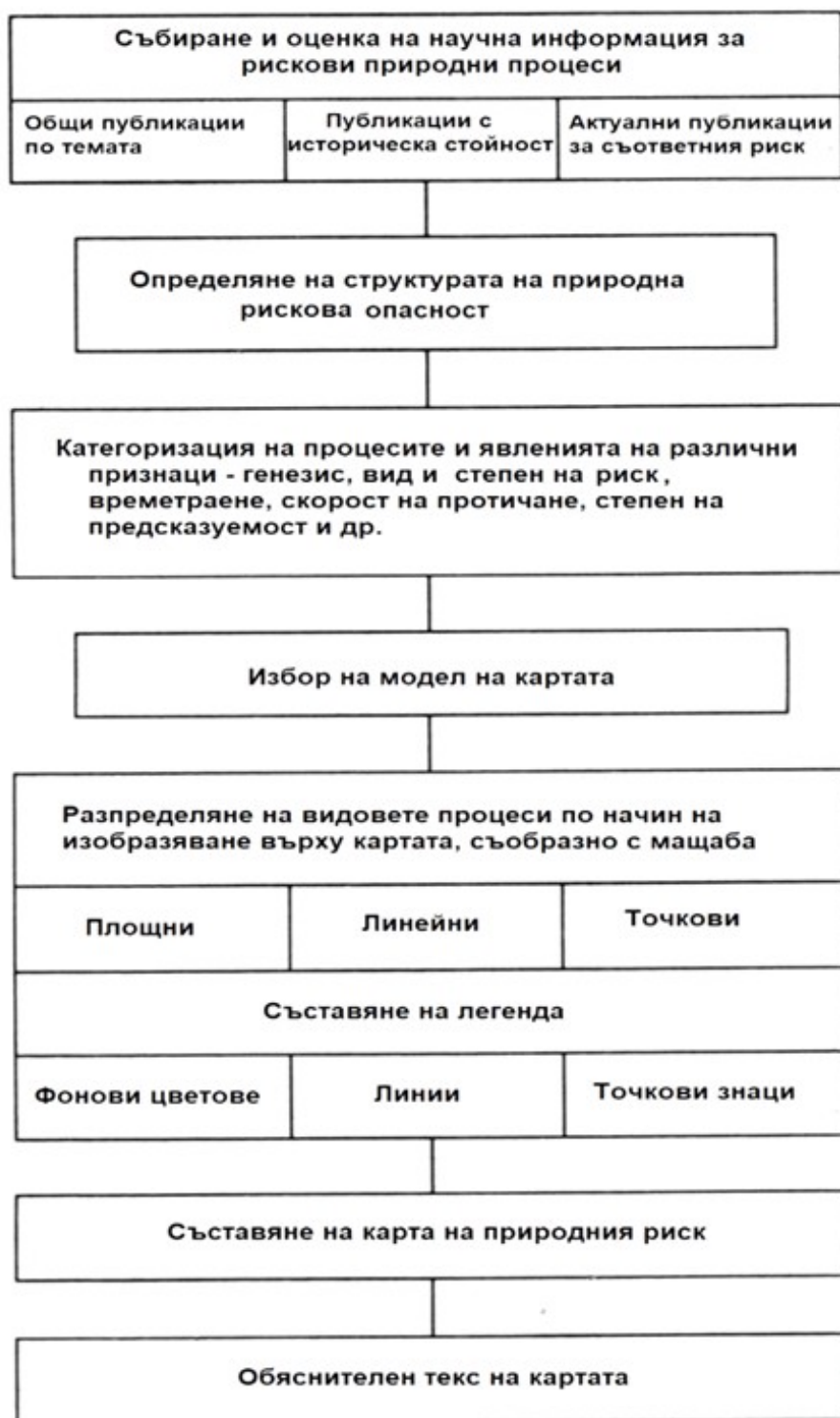
Фиг. 1. Алгоритъм за събиране на информация, анализ и картиране на природен риск
