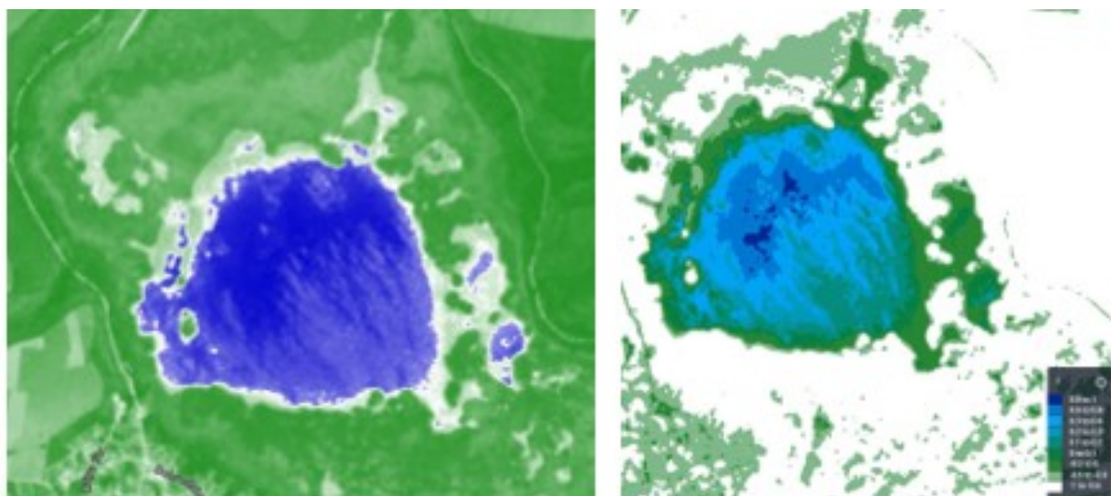
Фиг. 3. Пространствен модел на съвременното състояние на Сребърската система от влажни зони, представящ NDWI индекс на основата на сателитно изображение от Sentinel 2.
