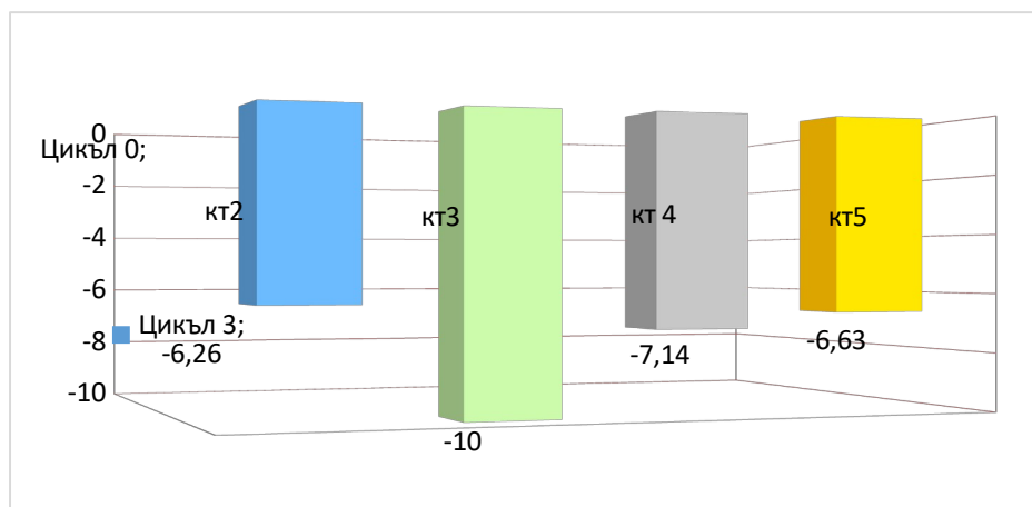
Фиг.7. Диаграма на вертикалните деформации между третия и нулевия цикъл
