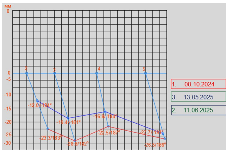
Фиг.6. Ходограма на хоризонталните деформации
