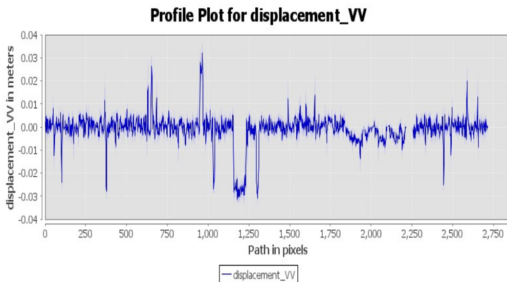
Фиг. 6. Теренен профил
