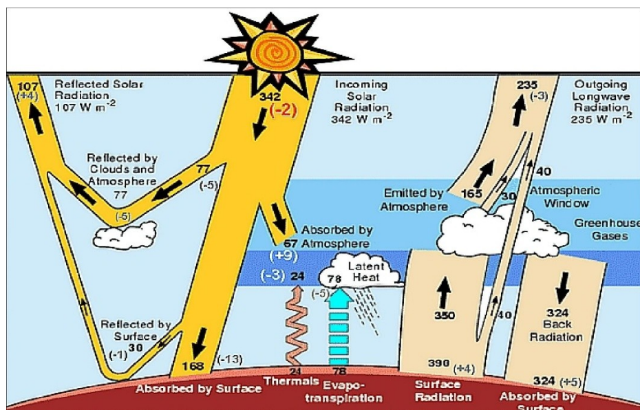
Фиг. 1. Схематично представяне на глобалните енергийни потоци в системата Слънце – климат от Кийл и Тренбърт (Бюлетин на Американското метеорологично дружество, 1997)
