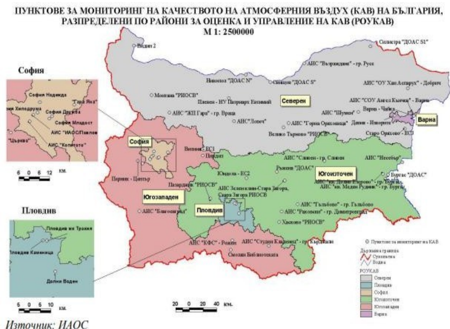
Фиг. 1. Райони за оценка и управление на КАВ и пунктове за мониторинг на КАВ
