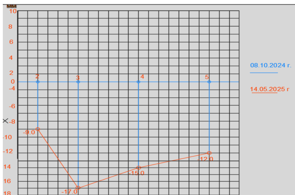
Фиг. 8. Ходограма на вертикалните деформации
